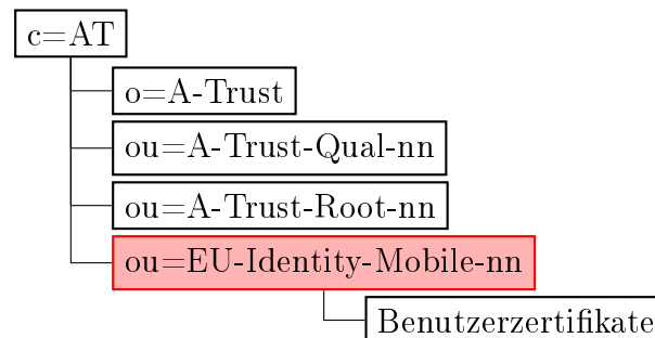
Abbildung 2: A-Trust Verzeichnisbaum
